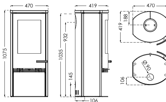
Brennkammer B / T: 340 / 271 Gewicht in kg: 139 / 141
